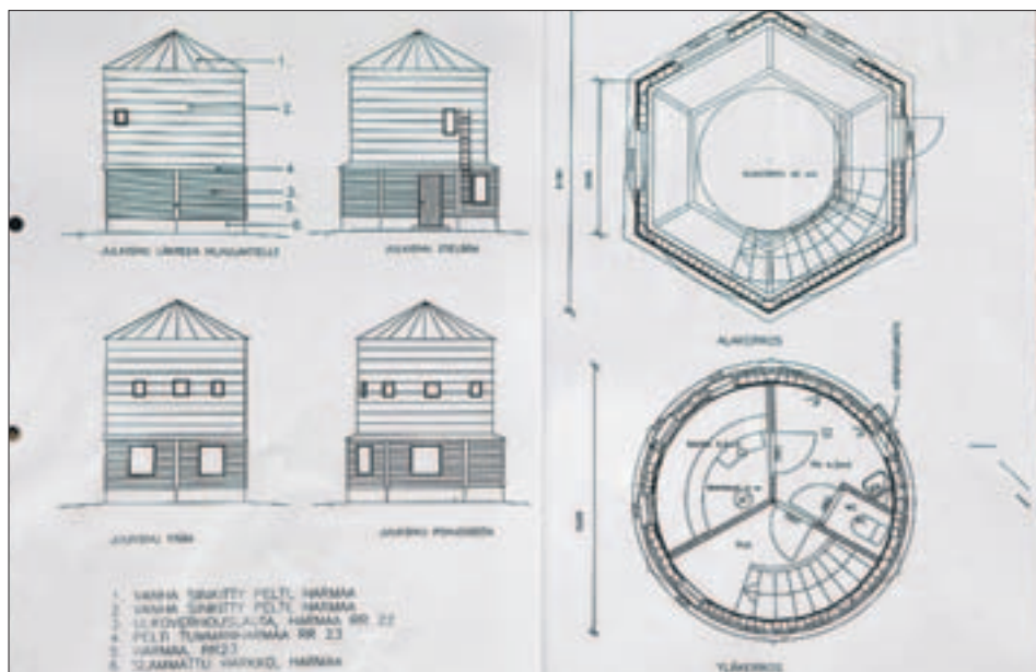
Pohjapiirustuksista näkee, millainen saunasta valmistuessaan tulee.
